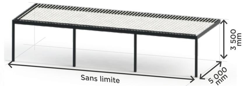
PergoToit Carport
