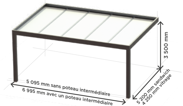
PergoToit Carport
