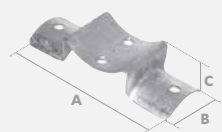
Connecteur pour bois ronds Réf. 94ACRGALCANN2R
